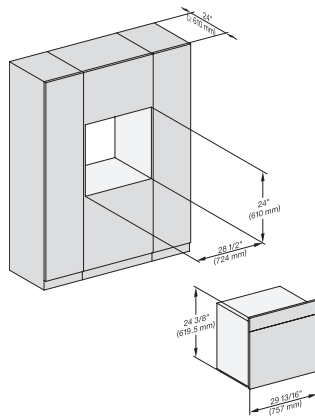
DGC7x8(X), Einbau, 30 Zoll, Proud, XXL
