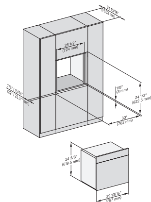
DGC7x8(X), Einbau, 30 Zoll, Flush inset, XXL
