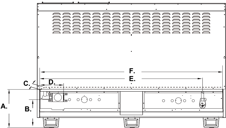
Modelo: FFSGS6187-60
