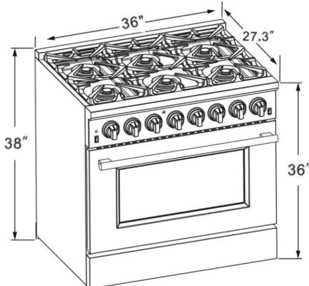
Model#: FFSGS6187-36
