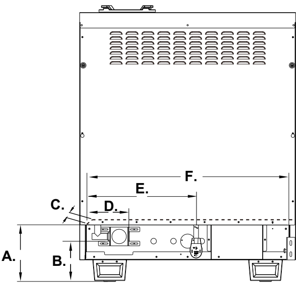
Modelo: FFSGS6187-30
