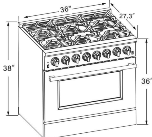
Modèle: FFSGS6187-36
