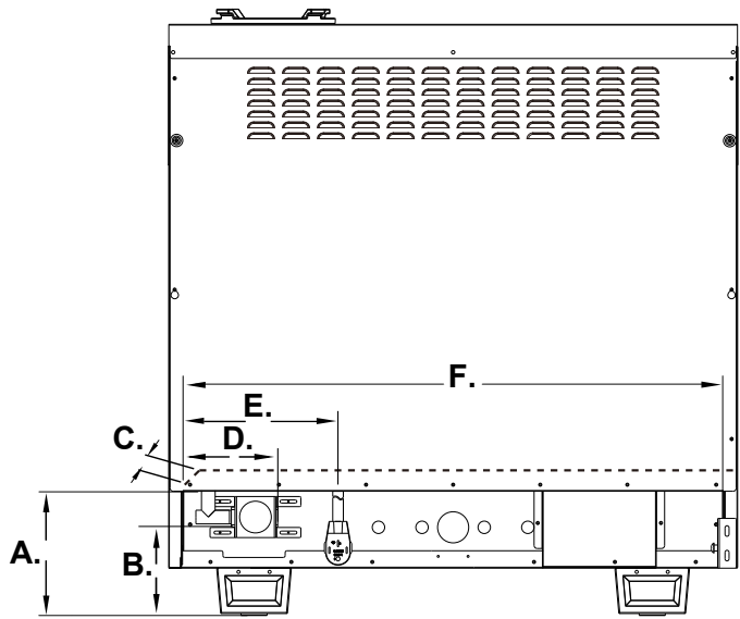
Modèle: FFSGS6187-36
