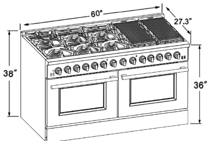
Modèle: FFSGS6187-60
