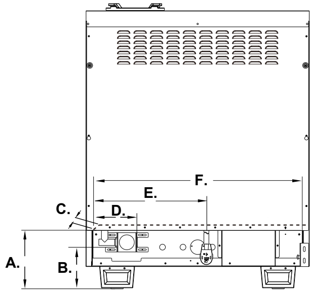
Modèle: FFSGS6187-30
