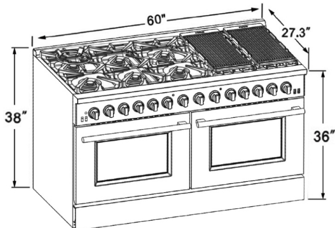
Model#: FFSGS6187-60
