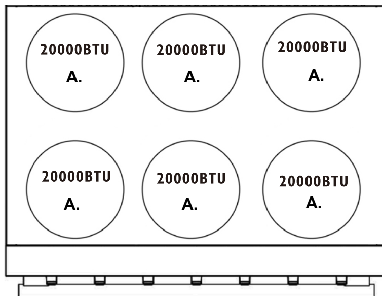
Modelo:FFSGS6187-36
