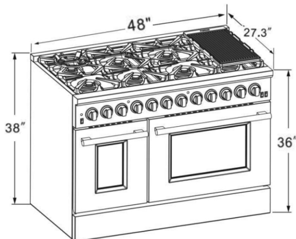
Model#: FFSGS6187-48
