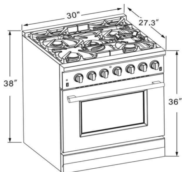
Model#: FFSGS6187-30
