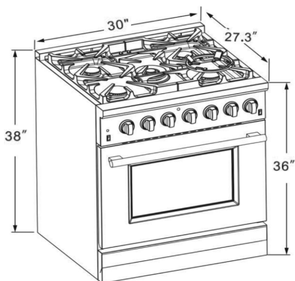
Modèle: FFSGS6187-30
