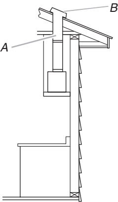
A. Conduit de dia. 6" (15,2 cm) pour décharge à travers le toit
