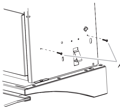
A. Vis de montage de 3,5 x 9,5 mm
