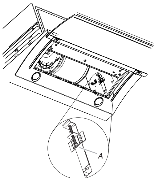
A. Vis T10 TORX®
