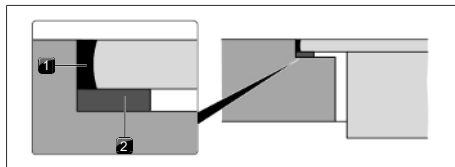
Fig. 11.13 Cinta selladora en caso de montaje enrasado
