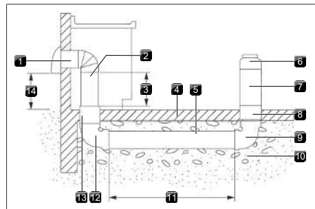
Fig. 11.19 Installations sur dalle de béton – évacuation murale
