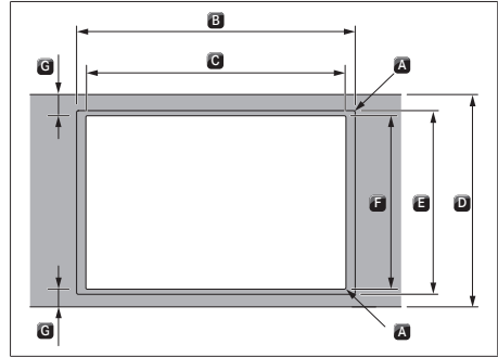
Fig. 11.8 Dimensiones de recorte para instalación enrasada
