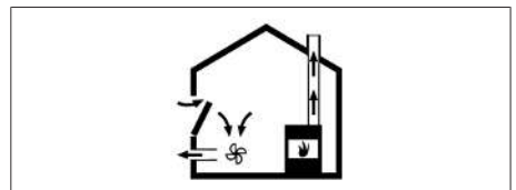
Fig. 11.2 Instalación de aire de escape – correcta
