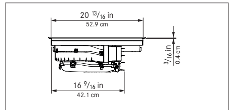
Fig. 5.6 Dimensiones del aparato vista lateral
