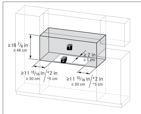
Fig. 11.3 Espacio necesario
