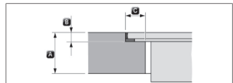
Fig. 11.5 Dimensiones de rebajo para instalación enrasada
