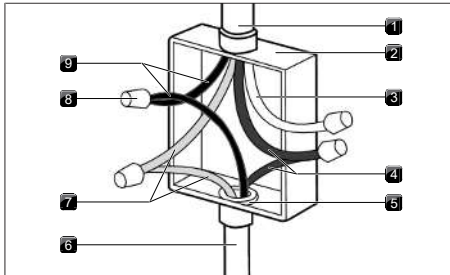
Fig. 11.20 Câble 4 fils
