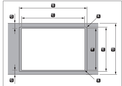
Fig. 11.4 Dimensiones de recorte para instalación enrasada
