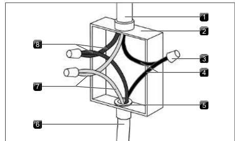
Fig. 11.21 Câble 3 fils
