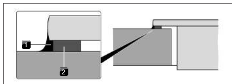
Fig. 11.12 Cinta selladora en caso de montaje superpuesto
