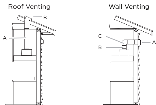
A. 8" (20.32 cm) round vent B. Wall cap
